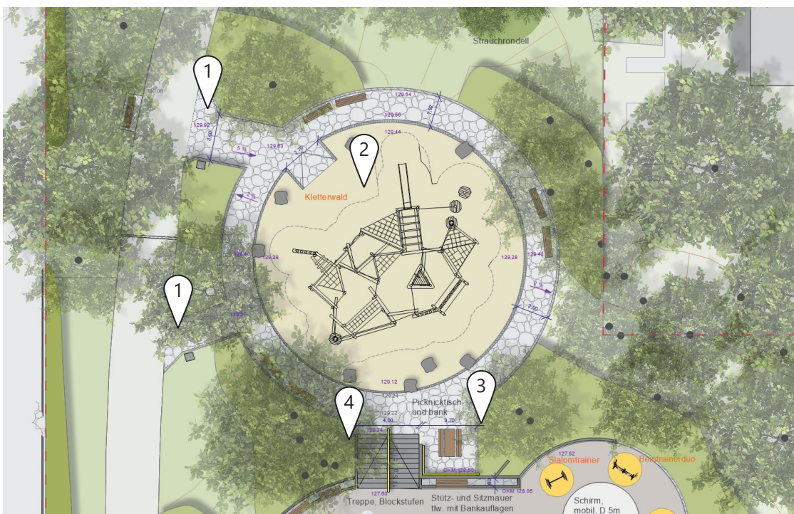
Oben: Schnitt Süd-Nord durch Sandrondell und Grosses Spielrondell Unten: Lageplan Grosses Spielrondell
