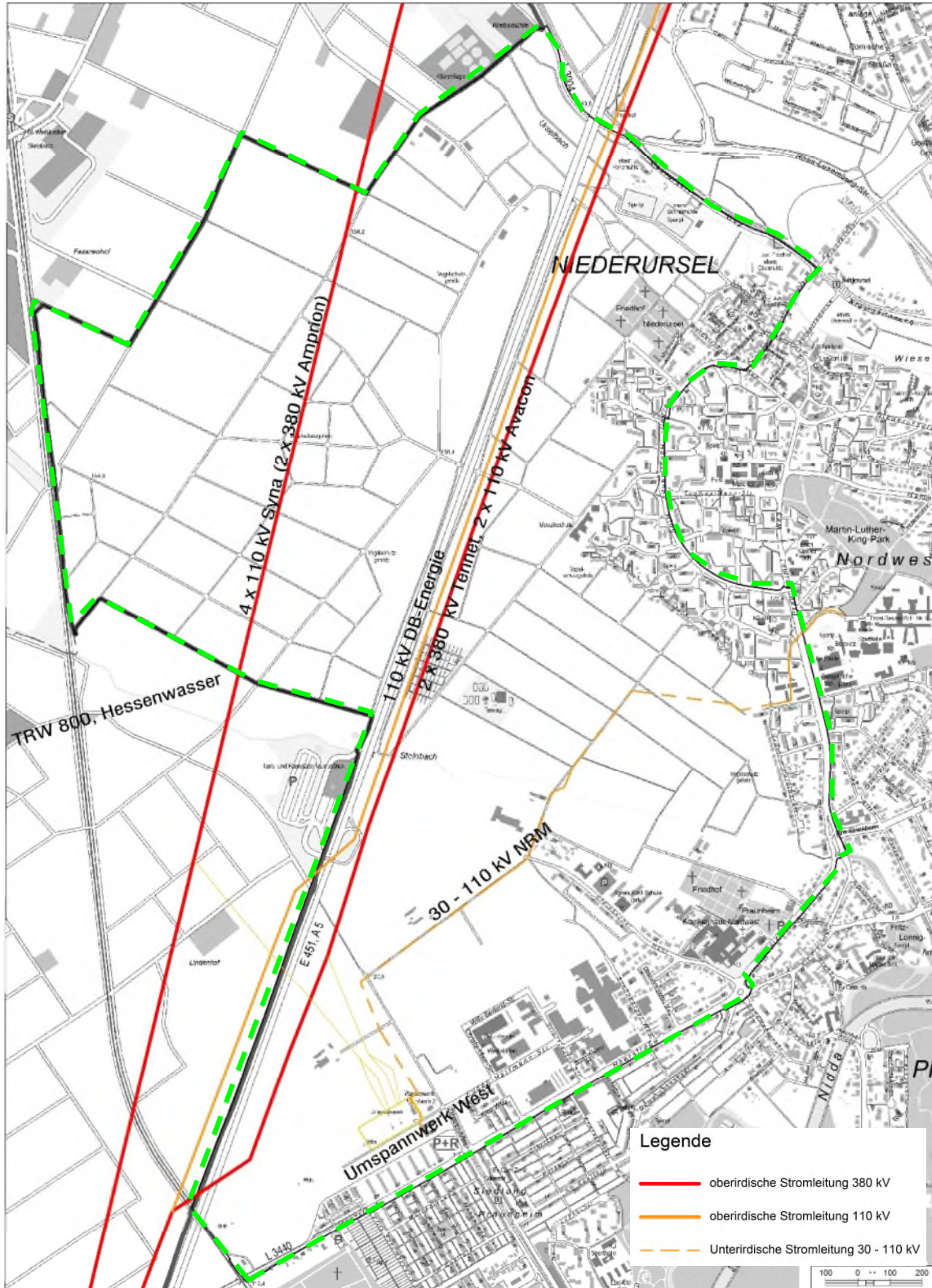
Abb. 3: Plangebiet des Stadtteils Frankfurt Nordwest (grün gestrichelt umrandet) mit Hoch- und Höchstspannungsleitungen, Umspannwerk West und Erdkabeltrasse
