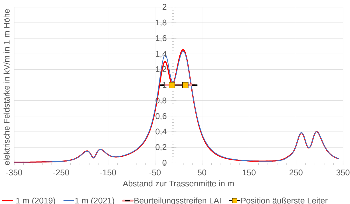
Abb. 16: Querprofil in 1 m Höhe zur TenneT / Avacon-Freileitung sowie links der DB Energie-Freileitung und rechts dem Anschluss an das Umspannwerk West im südlichen Teil des Plangebiets
