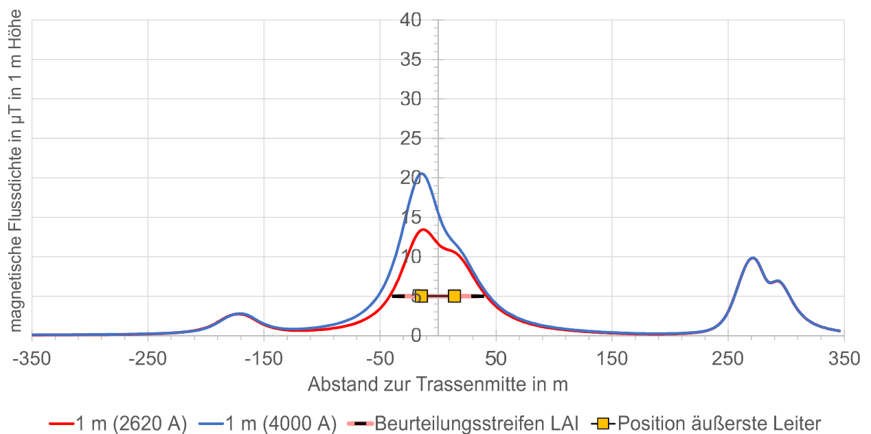
Abb. 10: Querprofil in 1 m Höhe zur TenneT / Avacon-Freileitung sowie links der DB Energie-Freileitung und rechts dem Anschluss an das Umspannwerk West im südlichen Teil des Plangebiets zur Verdeutlichung der schnellen Abnahme des Felds mit zunehmenden Abstand von der Leitungstrasse (keine Maximalwerte)
