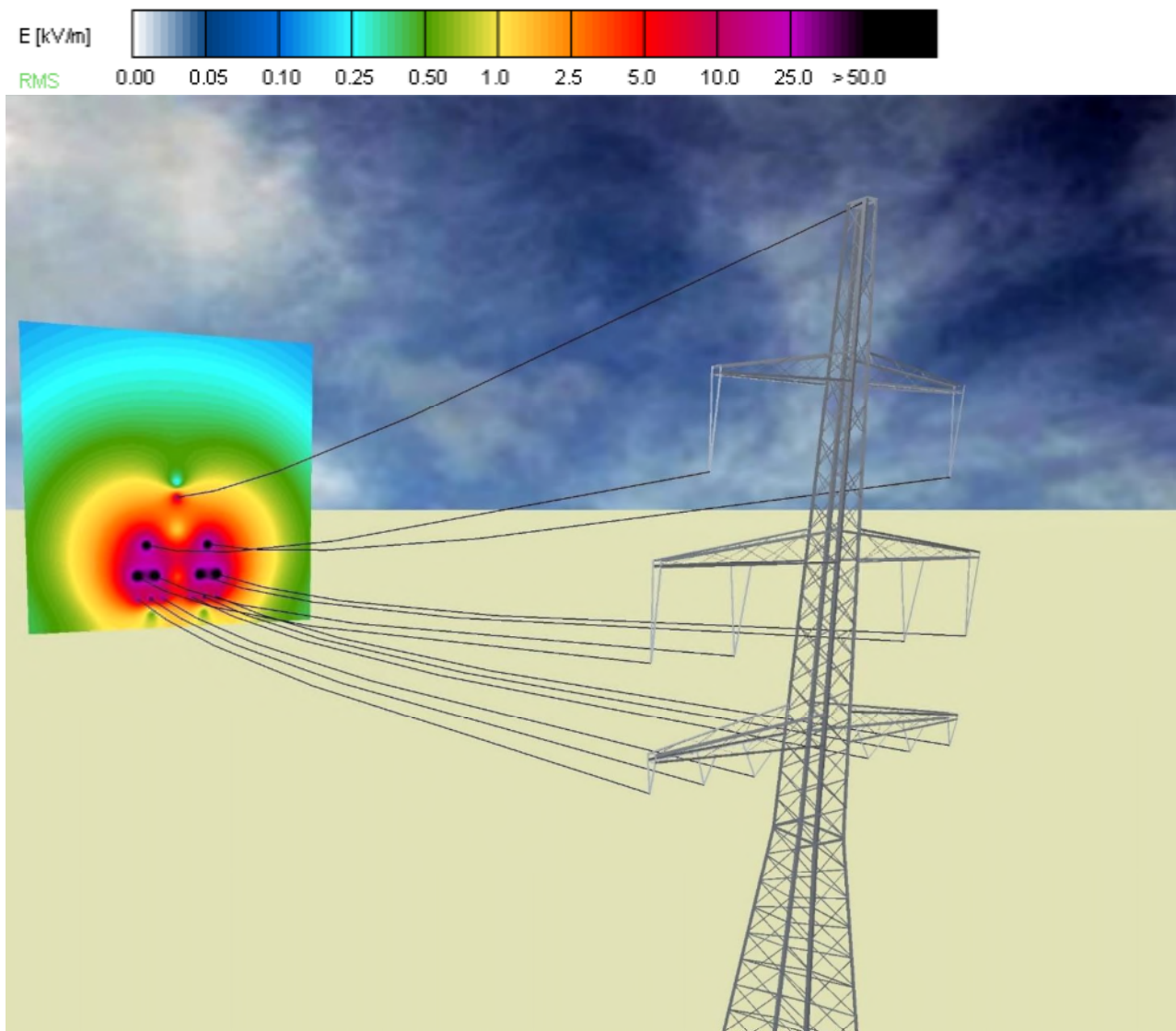
Abb. 19: Feldverteilung für die elektr. Feldstärke im vertikalen Schnitt im Bereich des größten Durchhangs durch die Amprion / Syna-Freileitung – geplante Konfiguration
