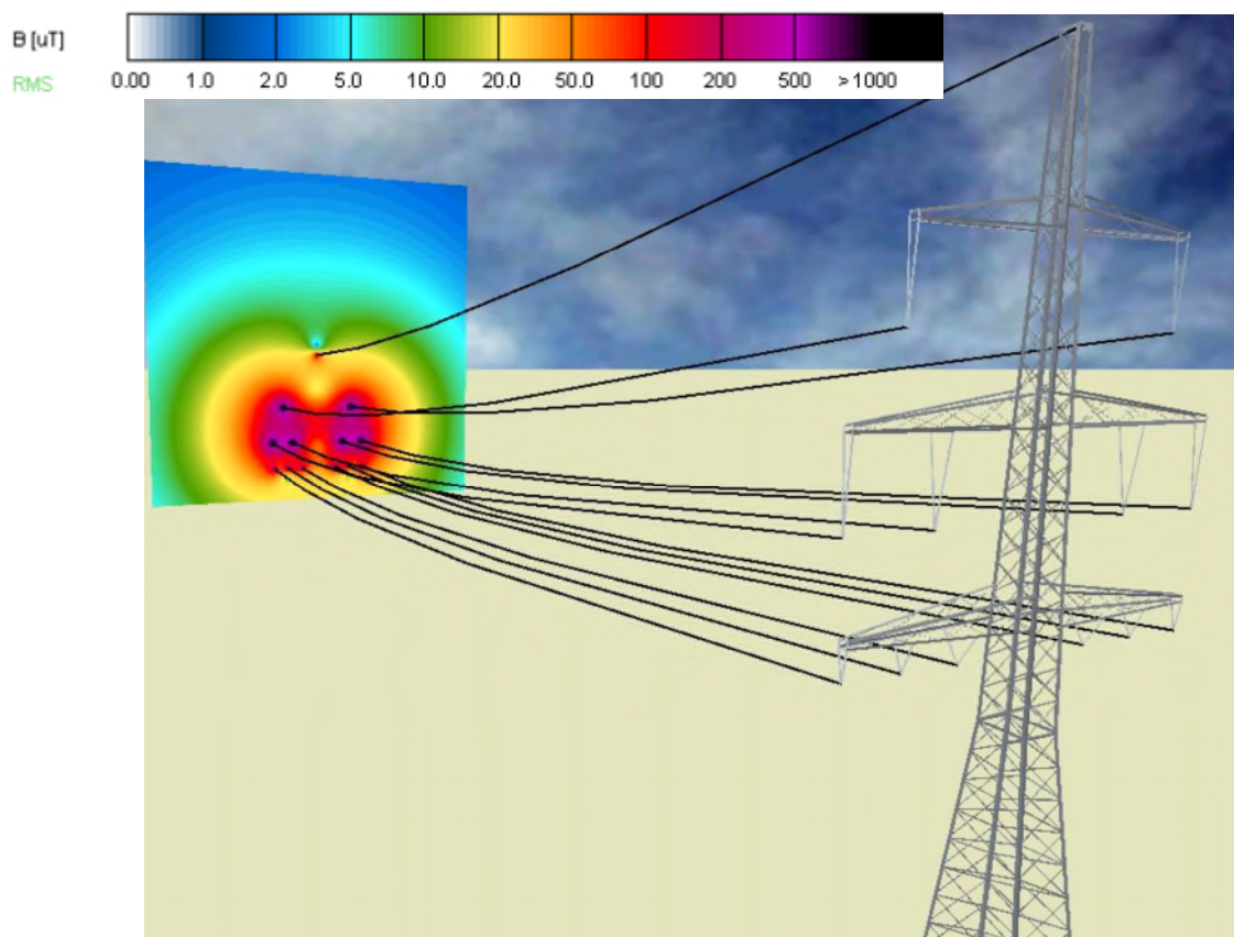
Abb. 17: Feldverteilung für die magnetische Flussdichte im vertikalen Schnitt im Bereich des größten Durchhangs durch die Amprion / Syna-Freileitung – Konfiguration nach Planung von Amprion
