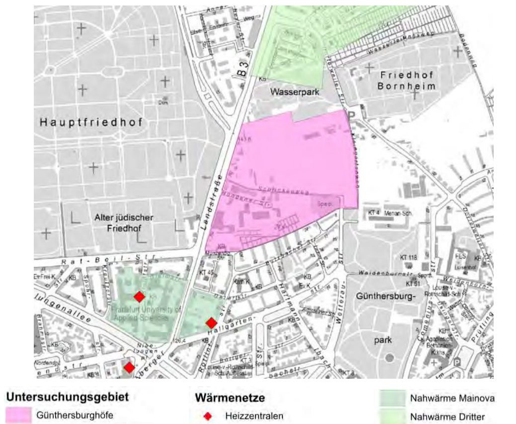
Abb. 55: Kartenauszug aus dem Abwärmekataster mit dem Geltungsbereich des Bebauungsplans B880 sowie dessen Umgebung (Quelle: Energiereferat der Stadt Frankfurt, 2018).
