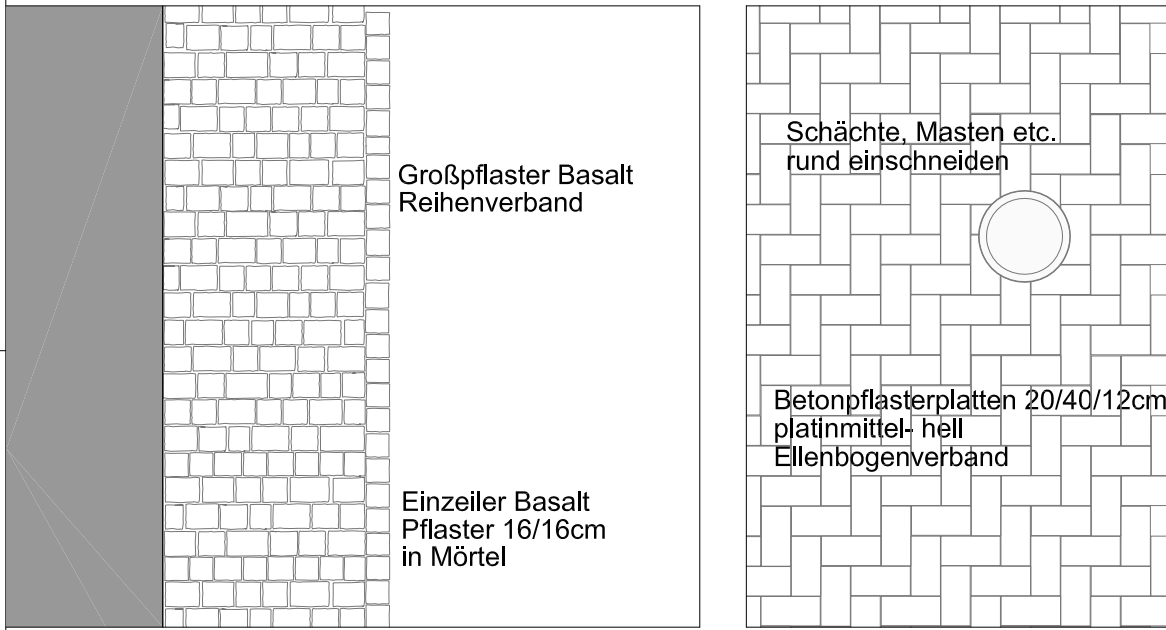
Traufstreifen Gebäude Betonbelag 1:50
