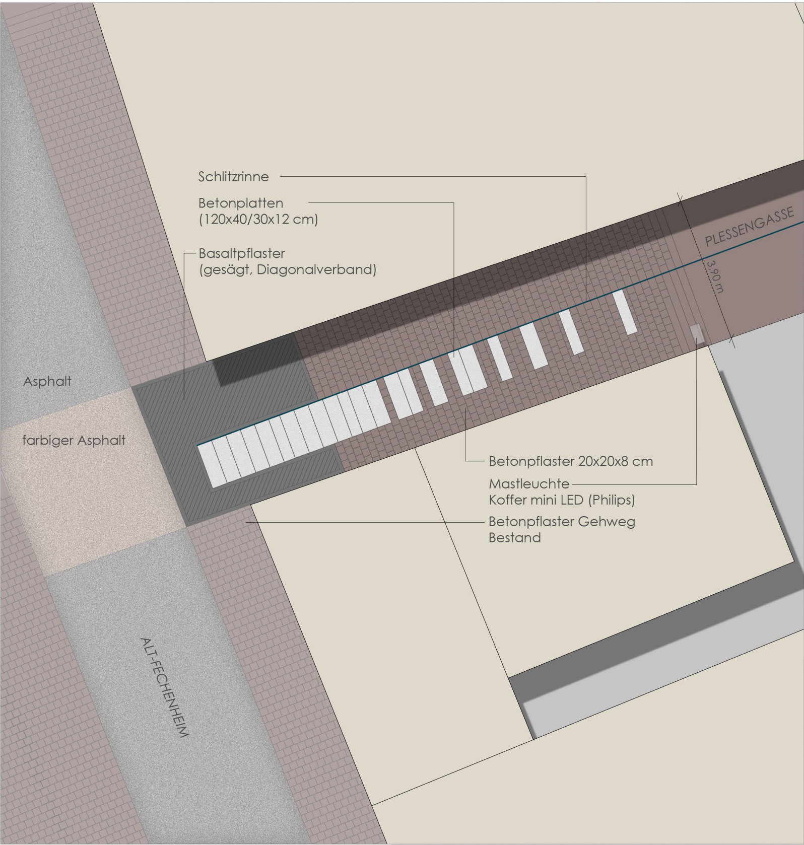
PLESSENGASSE - Mündungsbereich Alt-Fechenheim M 1:100
