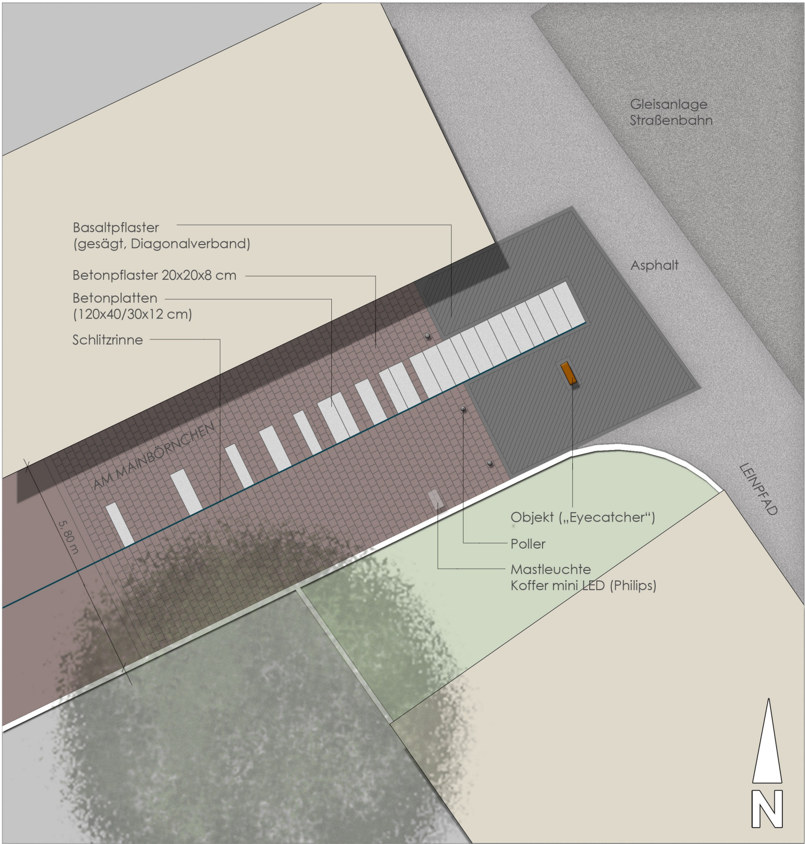
AM MAINBÖRNCHEN - Mündungsbereich Leinpfad / Mainufer M 1:100
