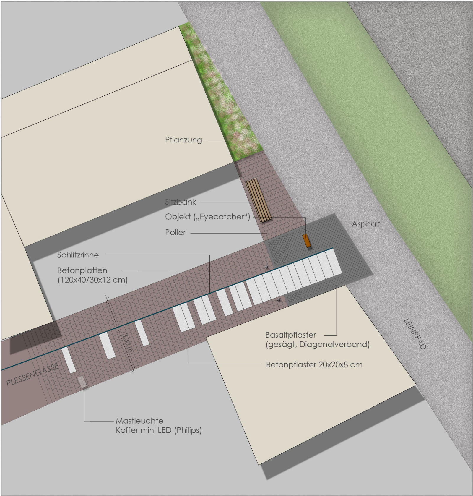
PLESSENGASSE - Mündungsbereich Leinpfad / Mainufer M 1:100
