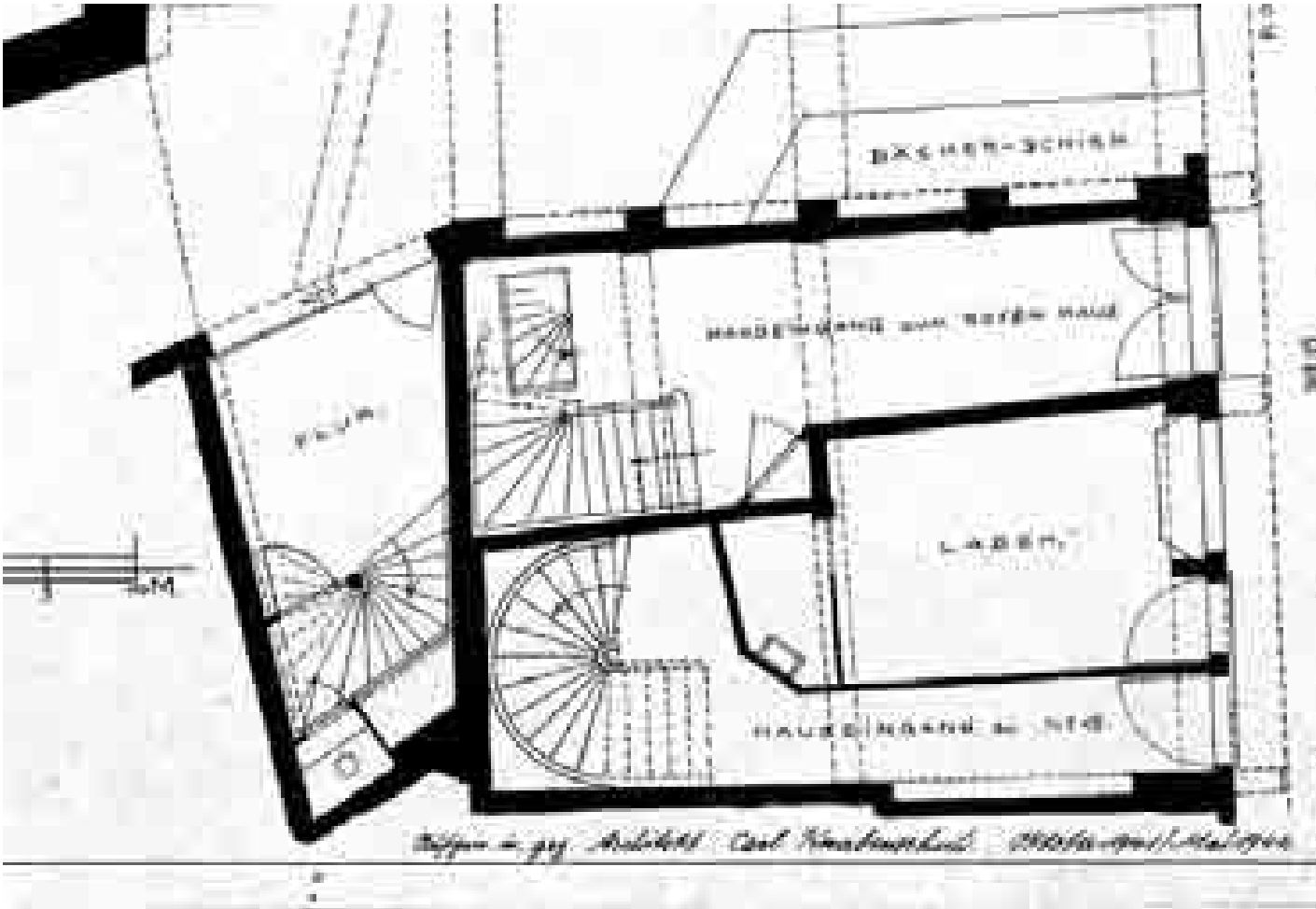
2 Erdgeschoss
