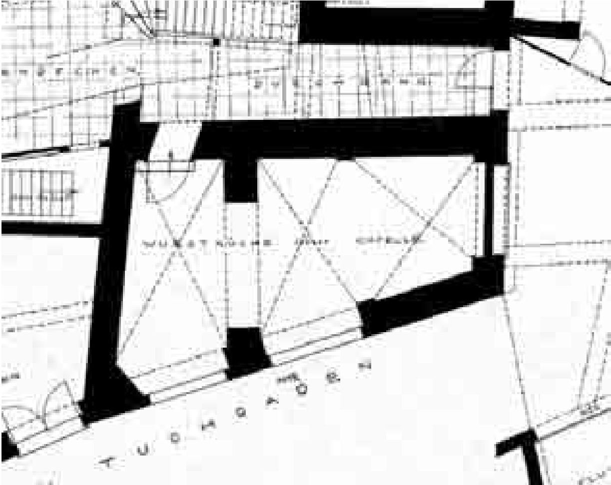
2 Erdgeschoss
