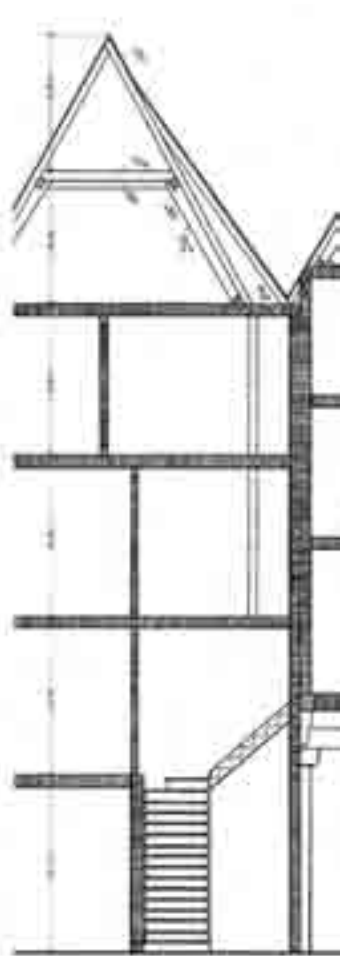
3 Schnitt
