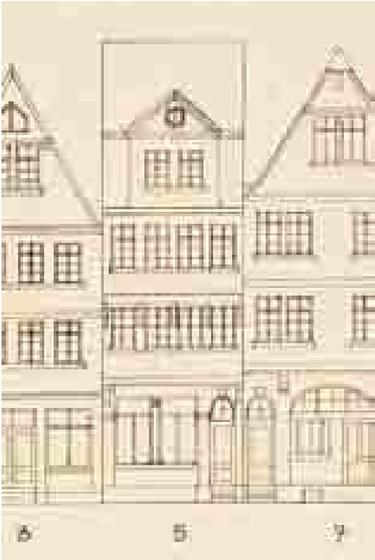
1 Nordansicht
