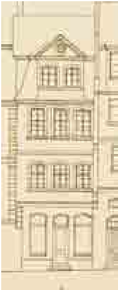
1 Ostansicht
