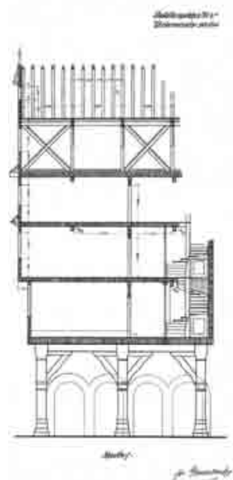
5 Schnitt Nord-Süd
