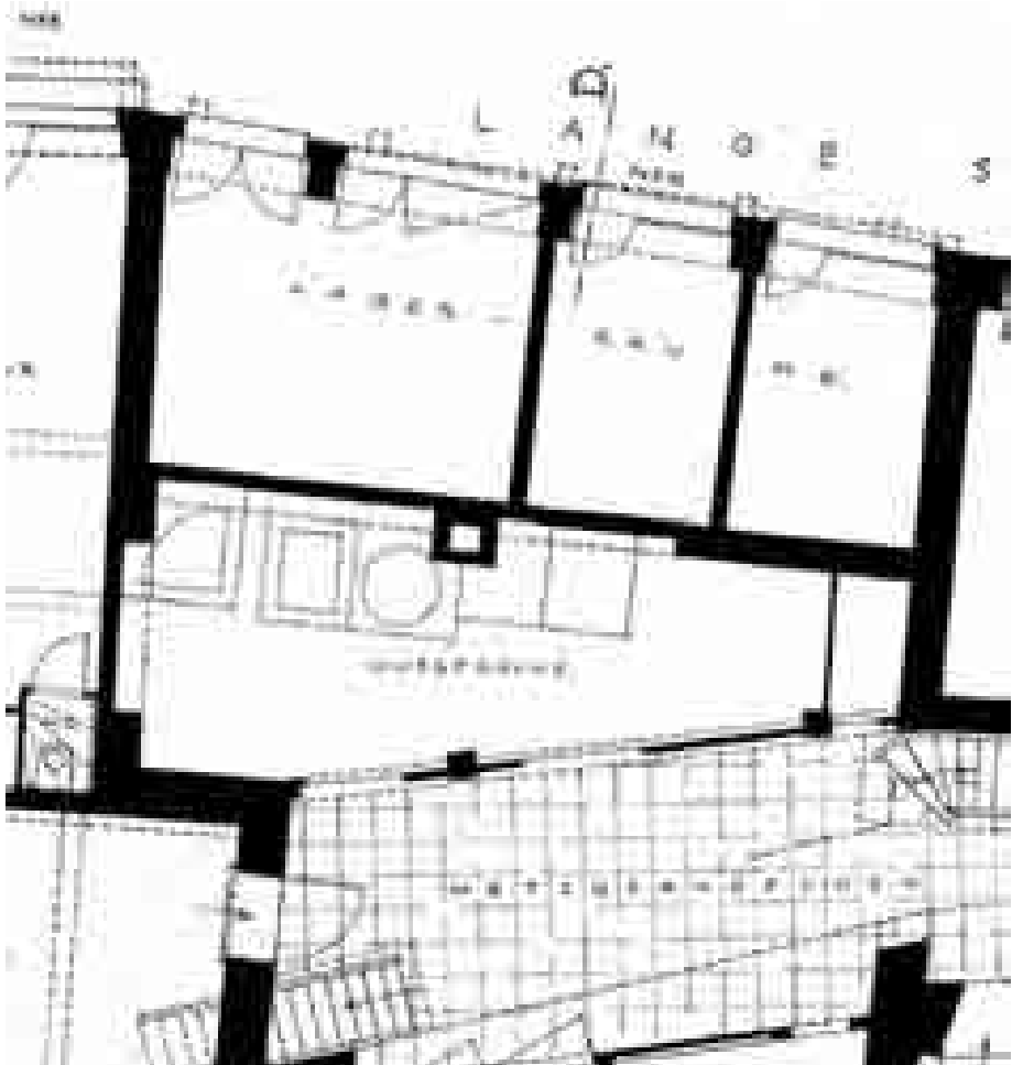
3 Erdgeschoss
