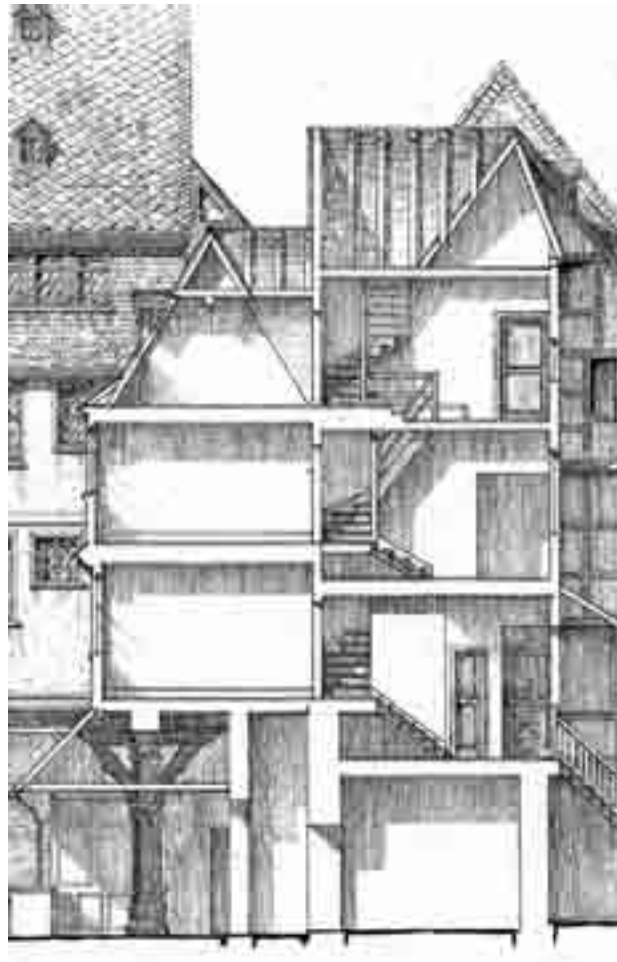
3 Schnitt Nord-Süd
