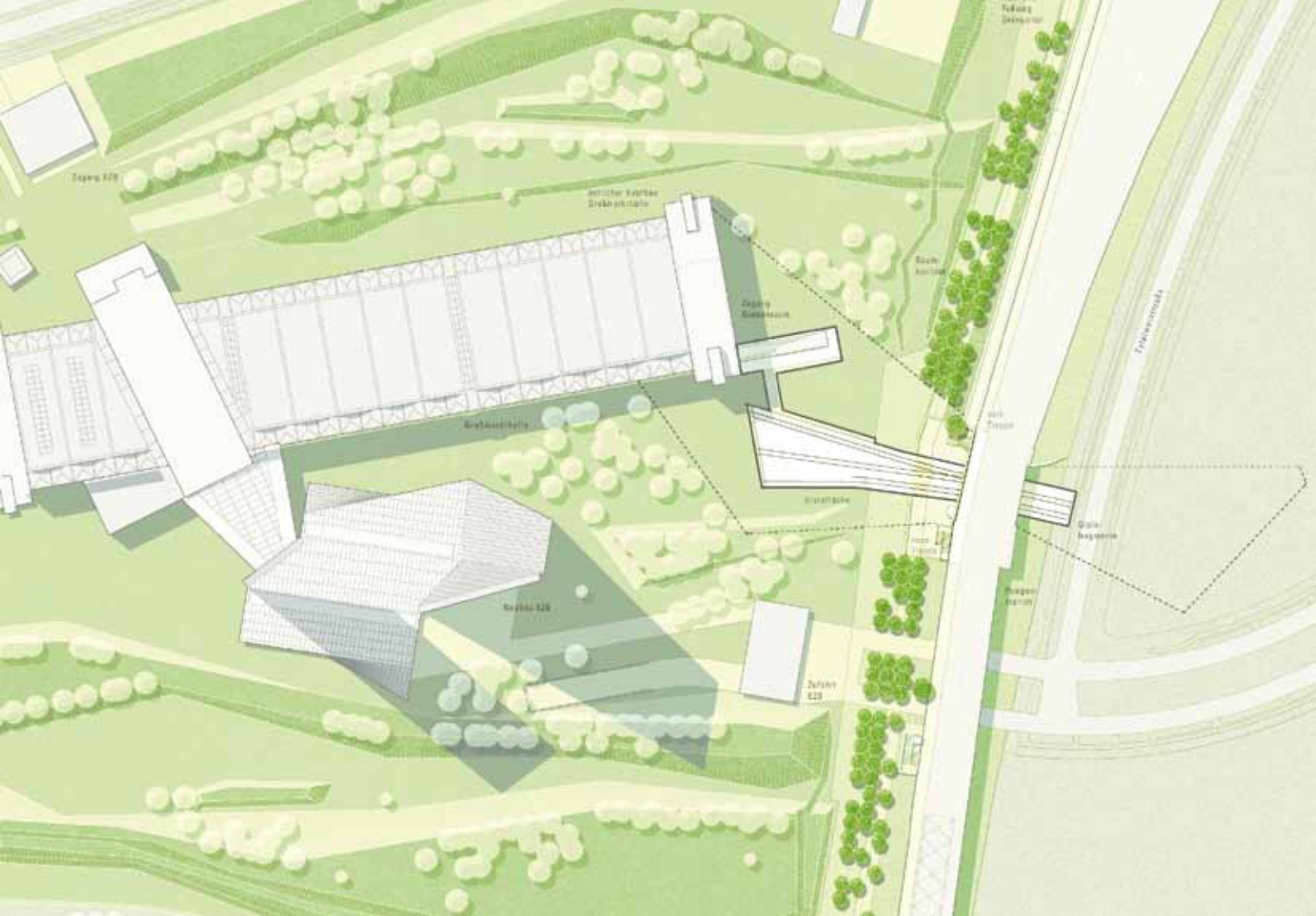
Lageplan
