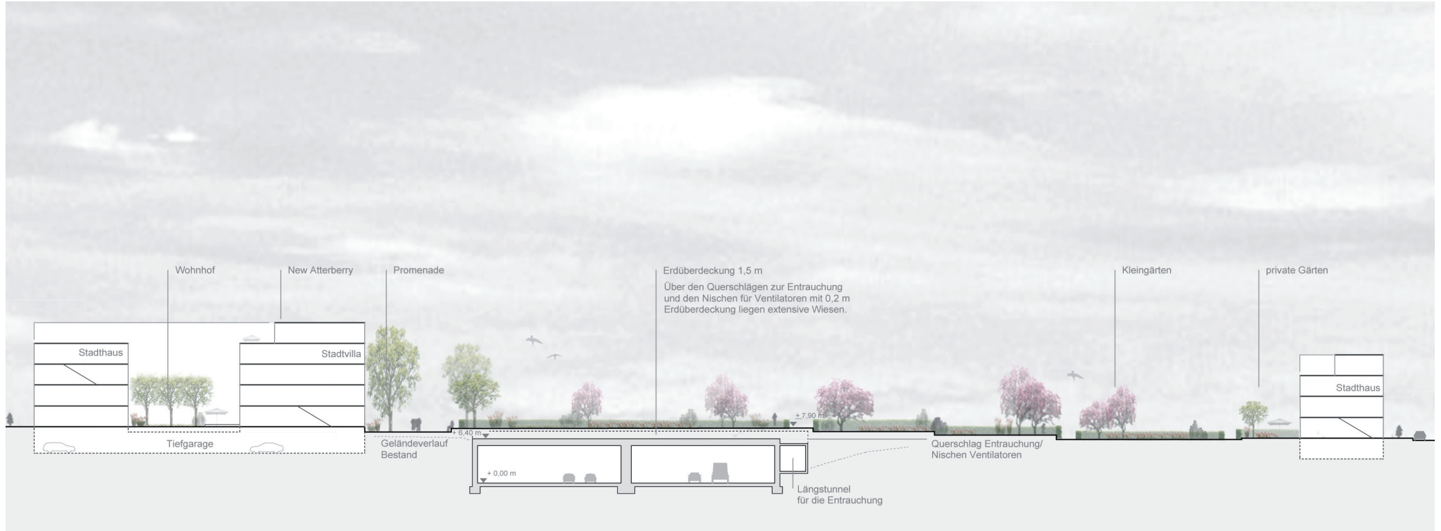
Schnitt Tunnelbauwerk zwischen New Atterberry und Festeburgsiedlung | M 1:500
